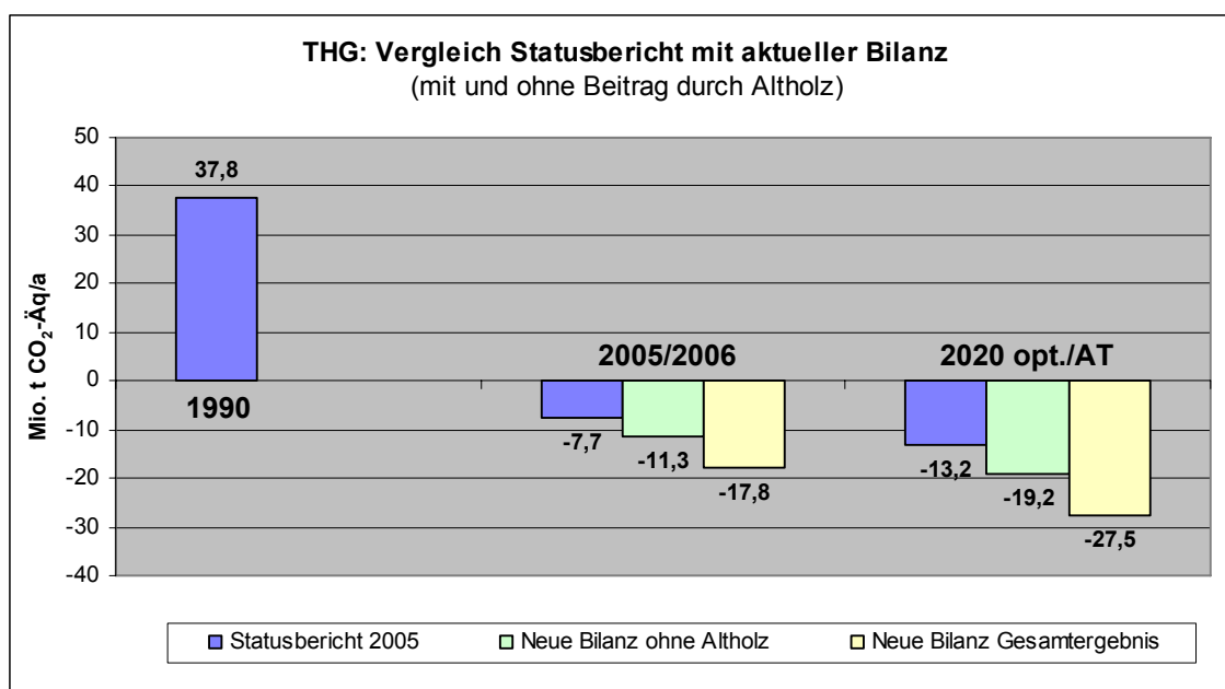
Abbildung 5.4 Gegenüberstellung der Gesamtergebnisse dieser Bilanz für THG (mit und ohne Altholz) zu Szenarien aus dem Statusbericht 2005 (Öko-Institut/IFEU 2005)
